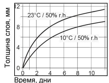
Диаграмма 1: скорость отверждения SikaTack®-MOVE IT .
